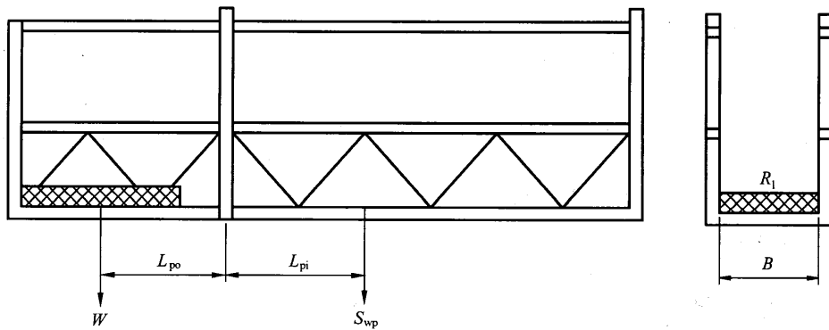
图6 悬臂平台
