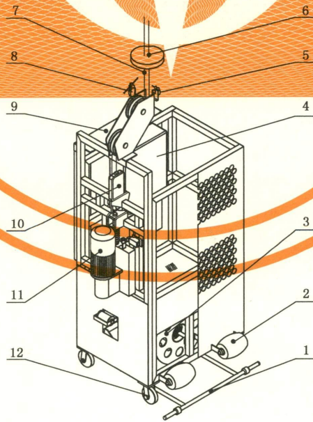
图2 双吊点平台
