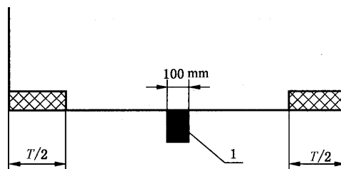
图 9 上升时遇突出物
