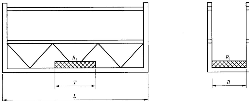
图 5 R_1 分布
